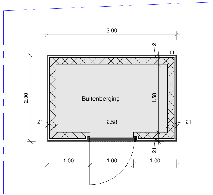
Grondplan
