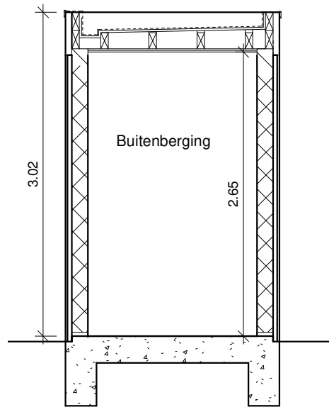
Doorsnede
