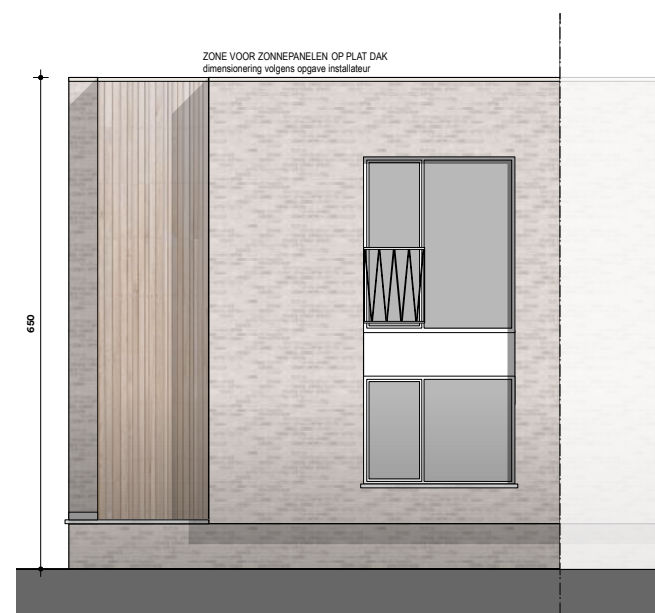
VOORGEVEL schaal 1/100
