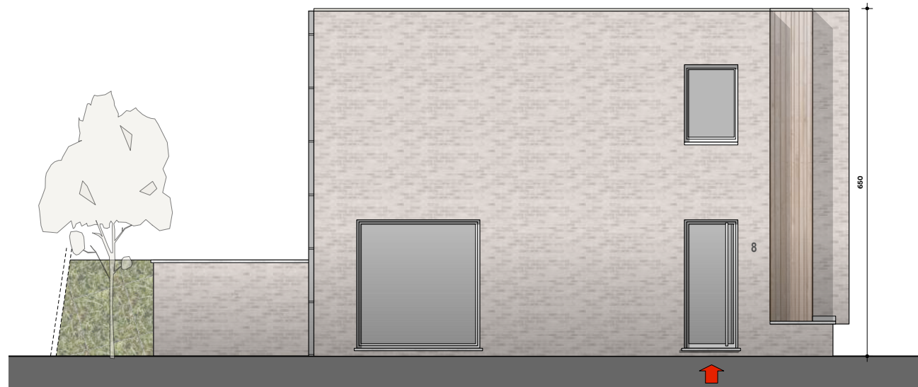
LINKERGEVEL schaal 1/100
