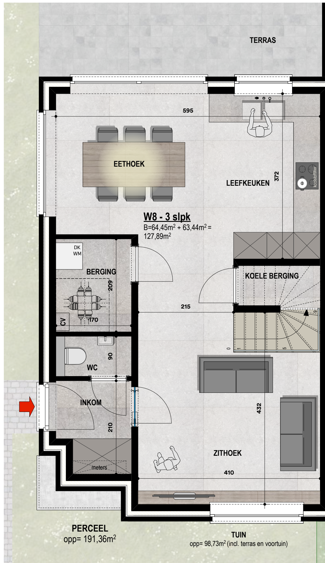
GELIJKVLOERS schaal 1/50
