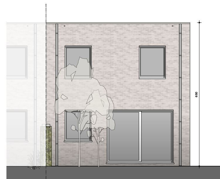
ACHTERGEVEL schaal 1/100
