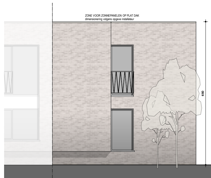
VOORGEVEL schaal 1/100
