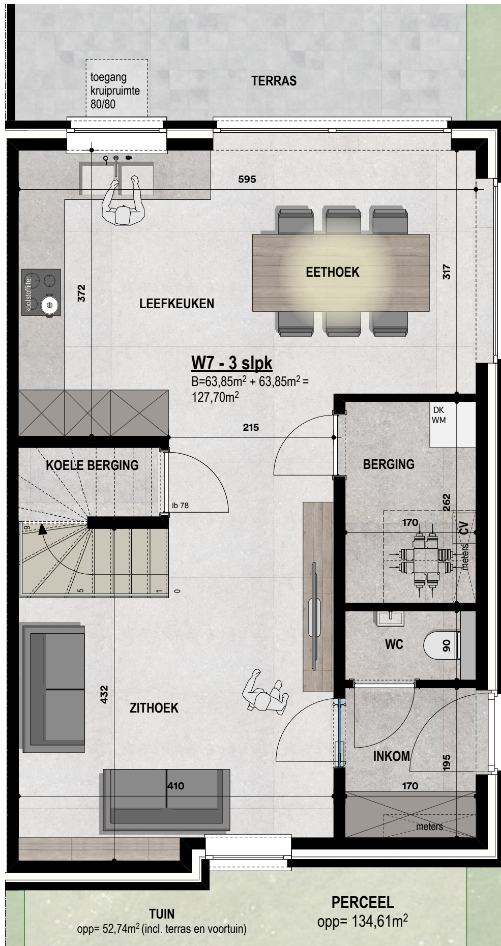
GELIJKVLOERS schaal 1/50
