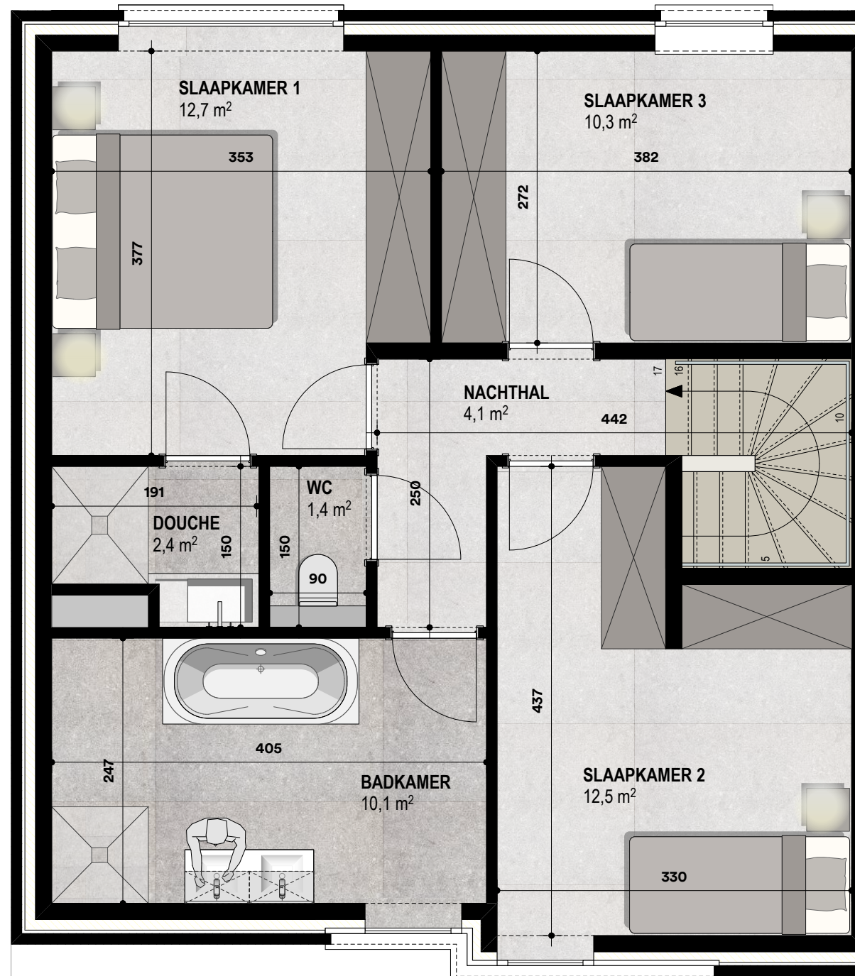
VERDIEPING schaal 1/50
