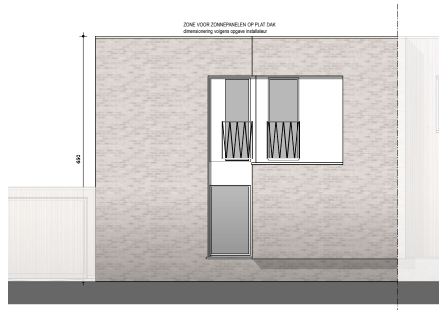
VOORGEVEL schaal 1/100
