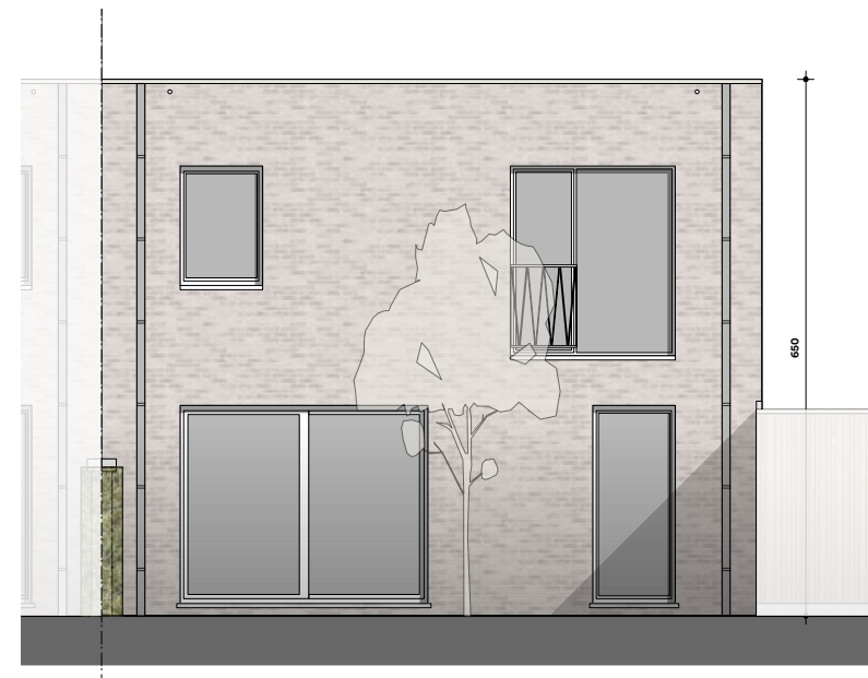
ACHTERGEVEL schaal 1/100
