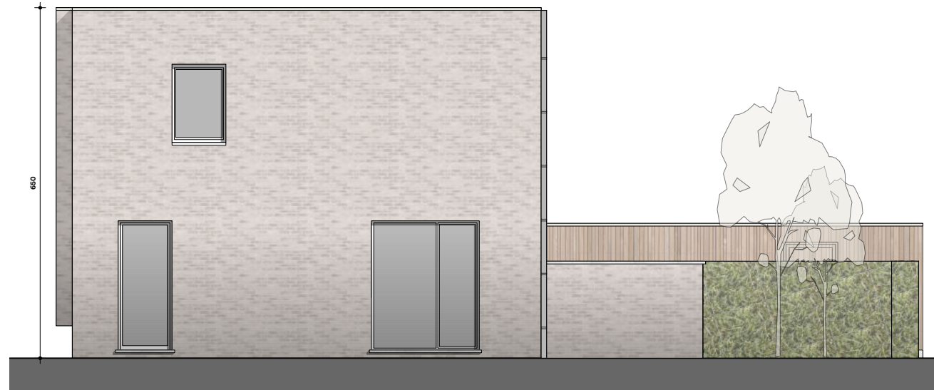
RECHTERGEVEL schaal 1/100
