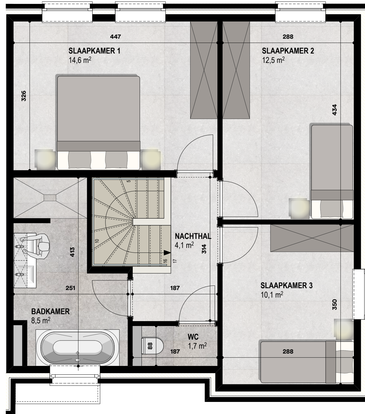
VERDIEPING schaal 1/50
