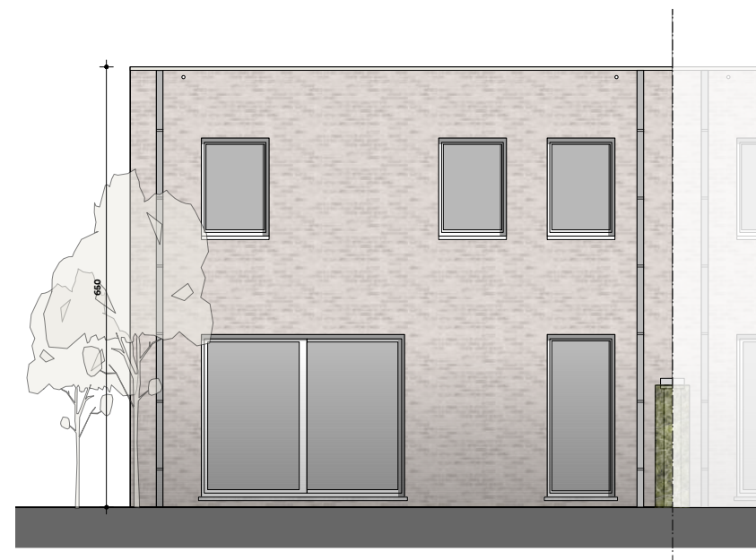
ACHTERGEVEL schaal 1/100
