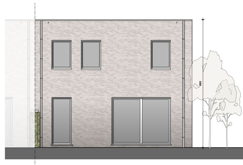
ACHTERGEVEL schaal 1/100
