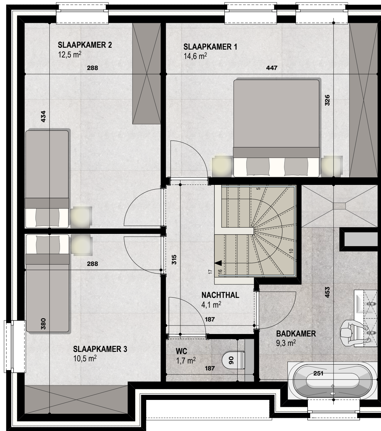
VERDIEPING schaal 1/50
