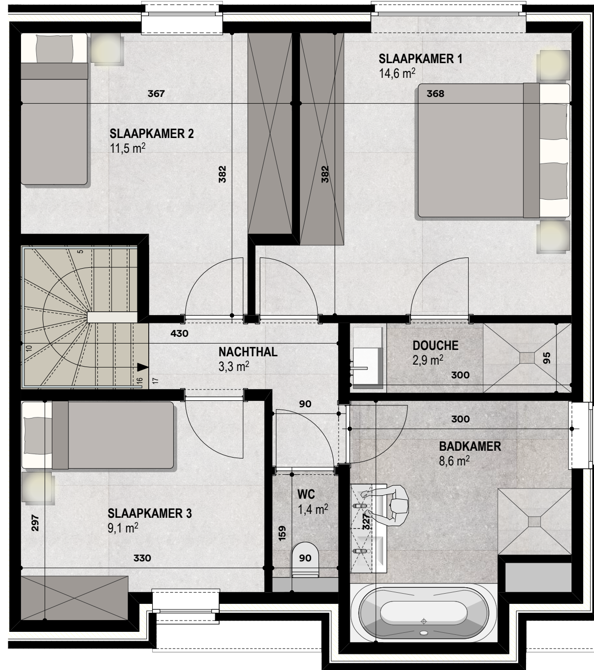
VERDIEPING schaal 1/50
