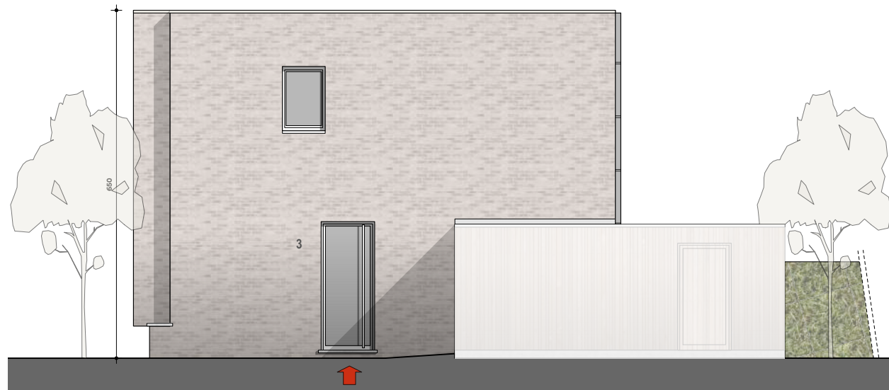
RECHTERGEVEL schaal 1/100
