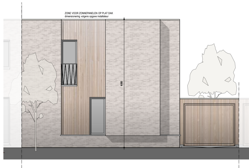
VOORGEVEL schaal 1/100
