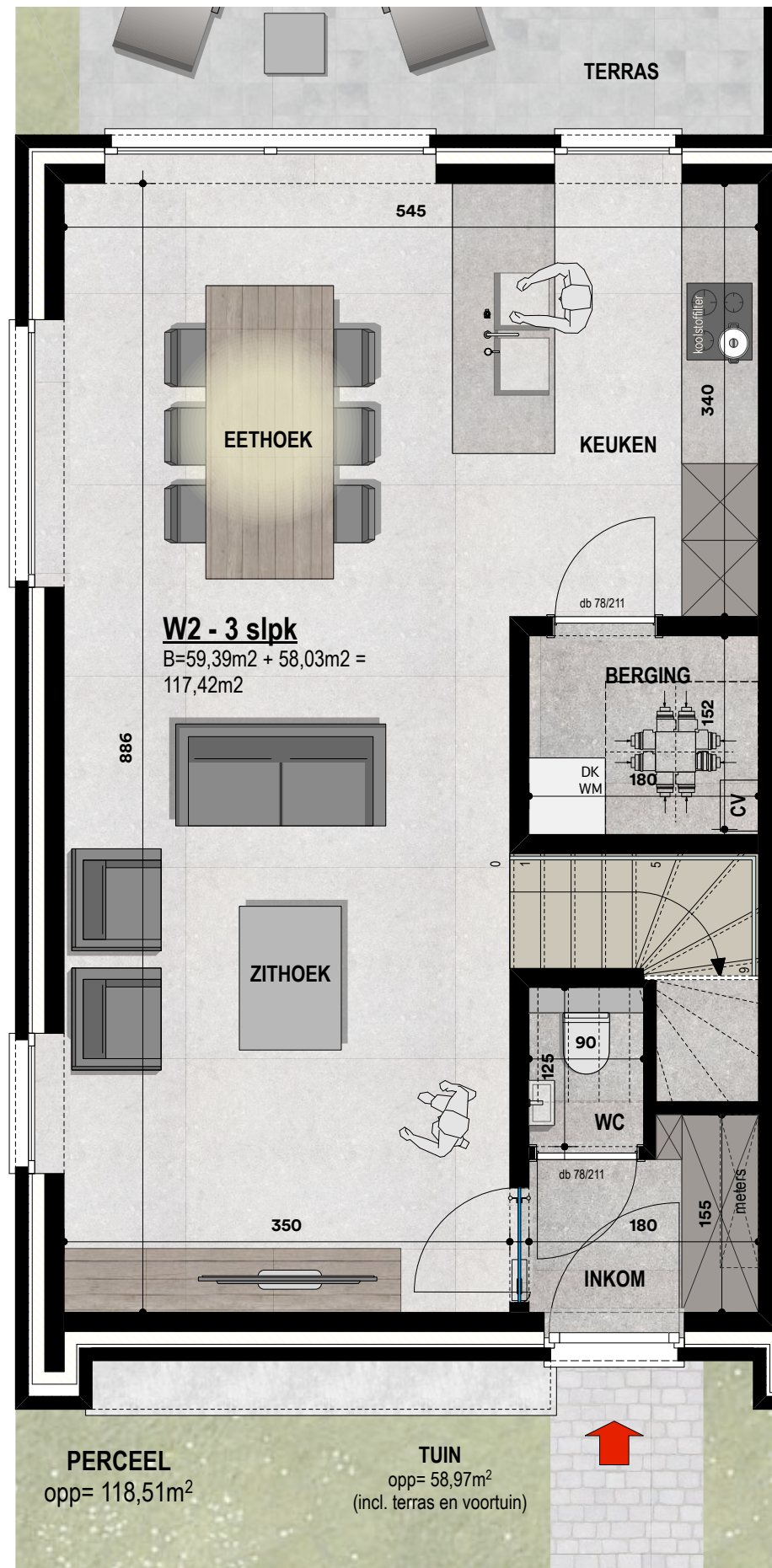
GELIJKVLOERS schaal 1/50
