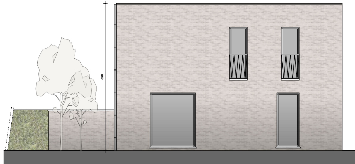
LINKERGEVEL schaal 1/100
