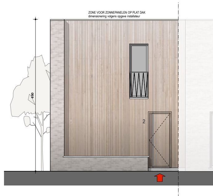
VOORGEVEL schaal 1/100
