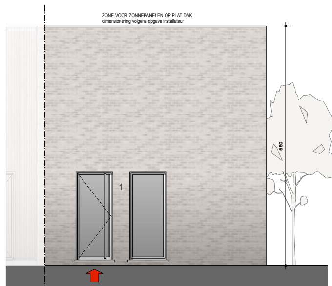
VOORGEVEL schaal 1/100
