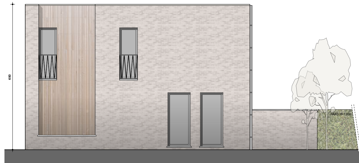
RECHTERGEVEL schaal 1/100
