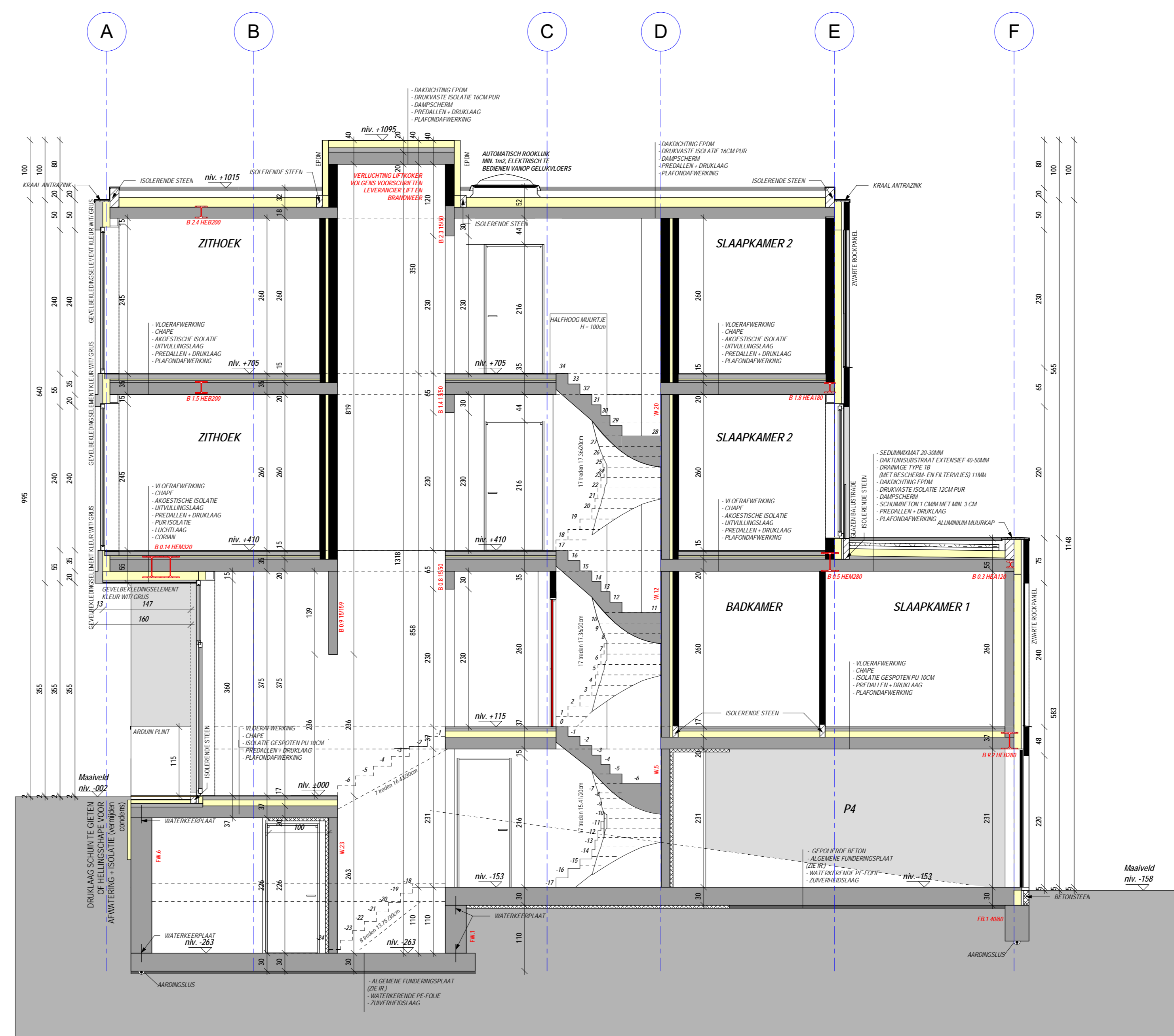
DOORSNEDE AA'
