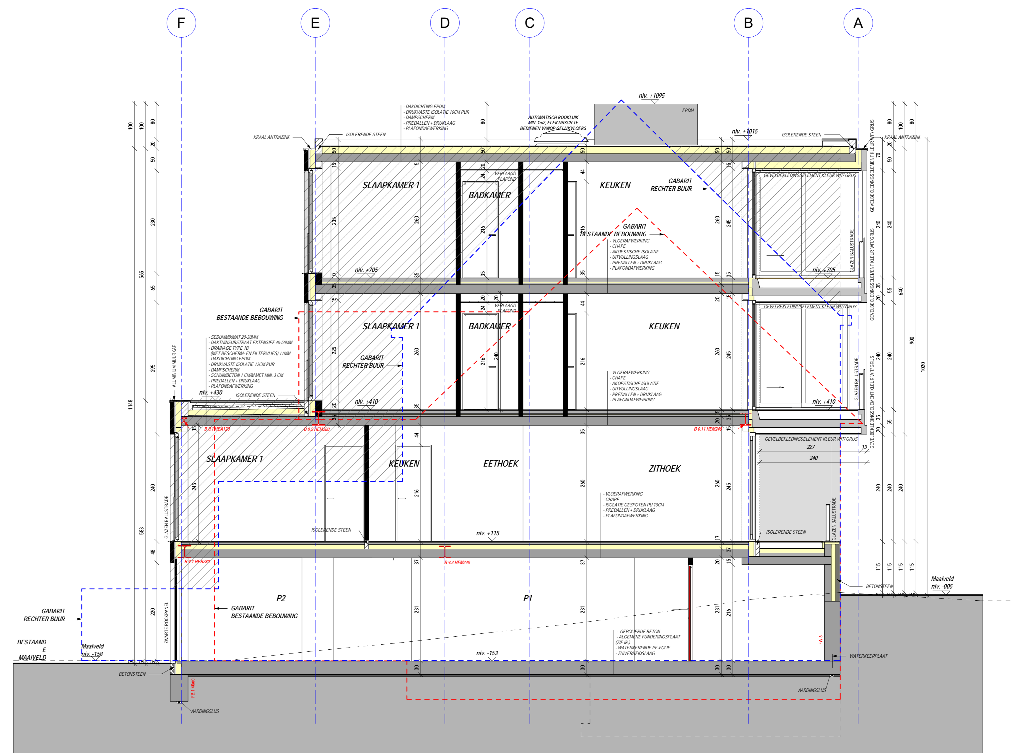
DOORSNEDE BB'
